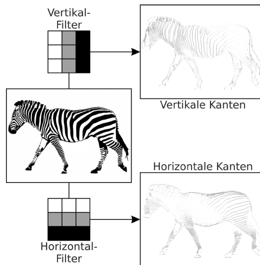
Abbildung 3: Auswirkungen verschiedener Filter Quelle: Creative Commons (CC0)
