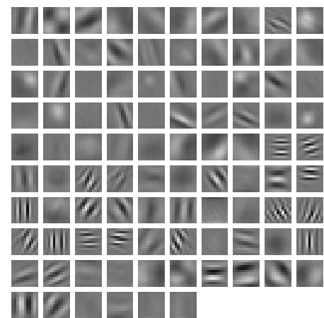
Abbildung 4: erlernte Filter der 96 Neuronen der ersten Schicht von AlexNet
